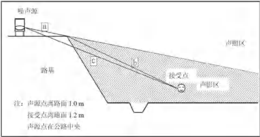
图 5.2-4 估计平均高度 h_m 的方法
